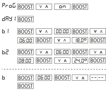
Obr. 3: Příklad programování
