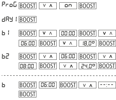
Rys. 3: Przykładowe programowanie
